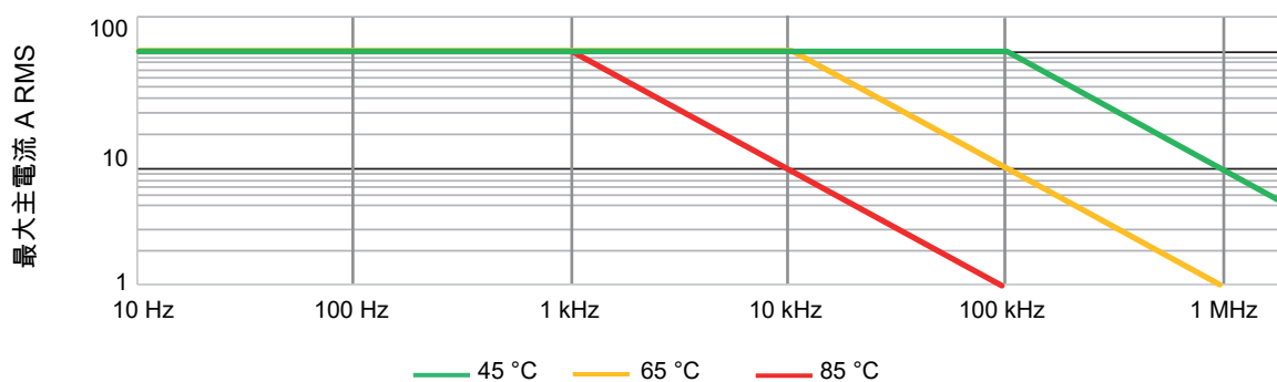
図 2: 周波数および周囲温度のディレーティング
