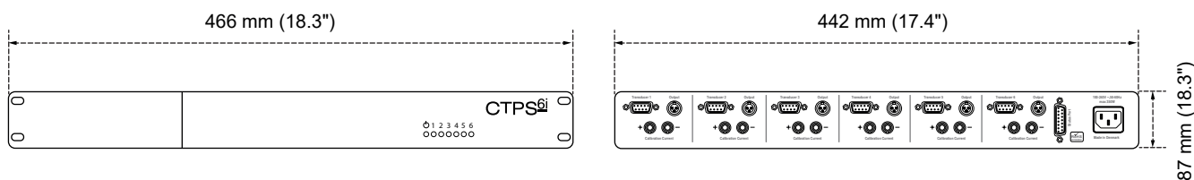
図 7: 寸法
