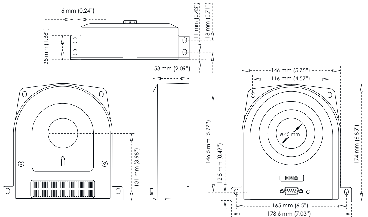
图 1.5: CTM1200ID/CTM1200ID-CD3000 尺寸
