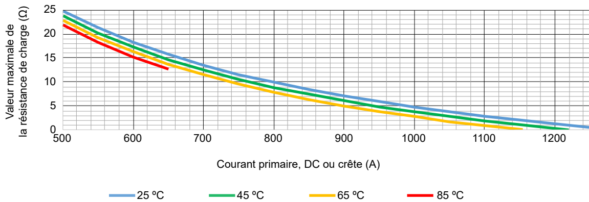
Figure 1.1 : Résistance de charge RM et limitation de la température ambiante
