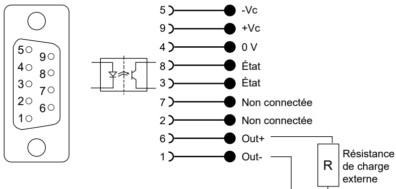
Figure 1.4 : Sortie de courant du D-SUB 9 broches standard
