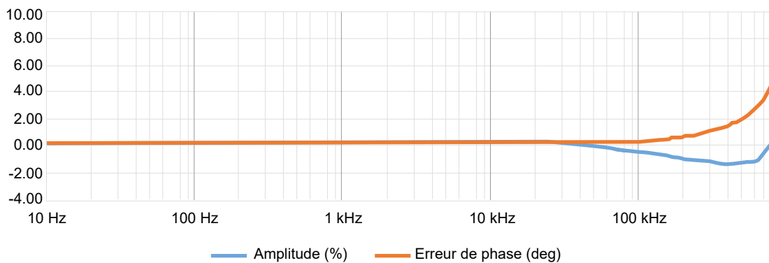
Figure 1.3 : Caractéristiques en fonction de la fréquence
