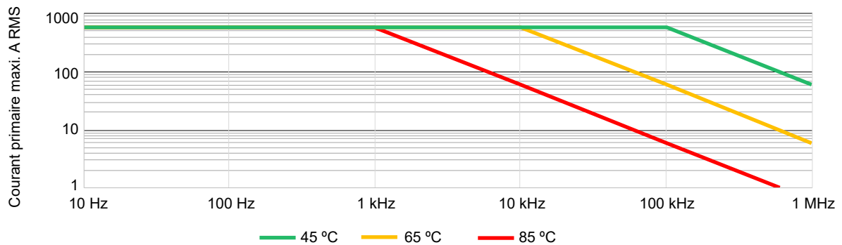
Figure 1.2 : Fréquence et limitation de la température ambiante
