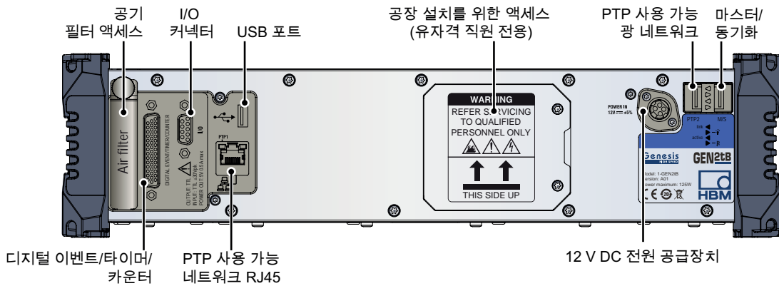
그림 9: 배면도 연결 개요
