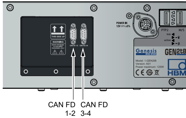
그림 29: GEN2tB, 설치된 CAN FD 상단 부분(세부) 포함
