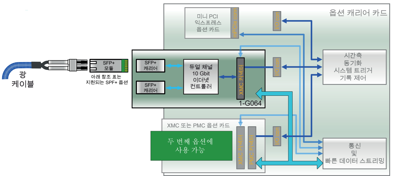
그림 20: 블록도 10Gbit 이더넷 카드, 광 (G081 필요)
