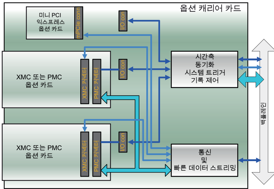
그림 19: 블록도 옵션 캐리어 카드
