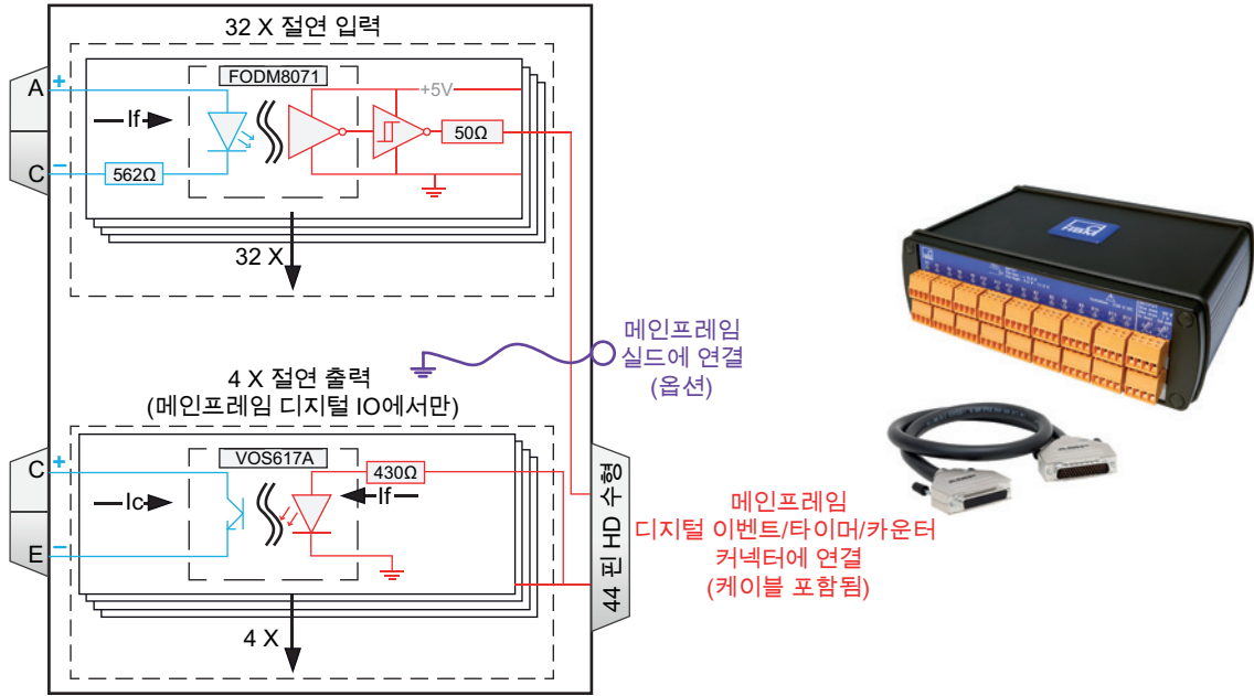
그림 26: 블록도 및 이미지
