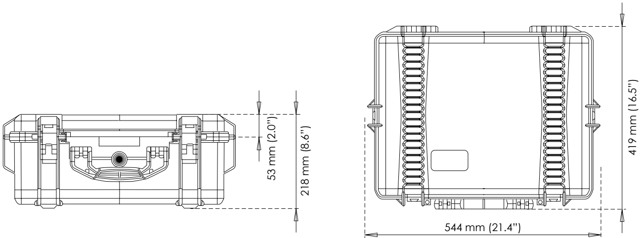
그림 34: 재활용 가능 하드커버 배송 케이스
