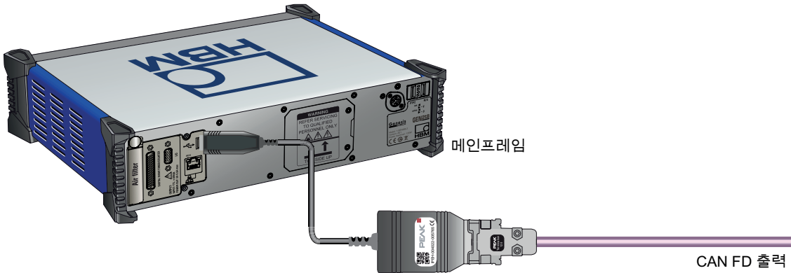
그림 31: GEN2tB 독립형 CAN FD 출력
