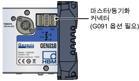
그림 12: 마스터/동기화 커넥터
