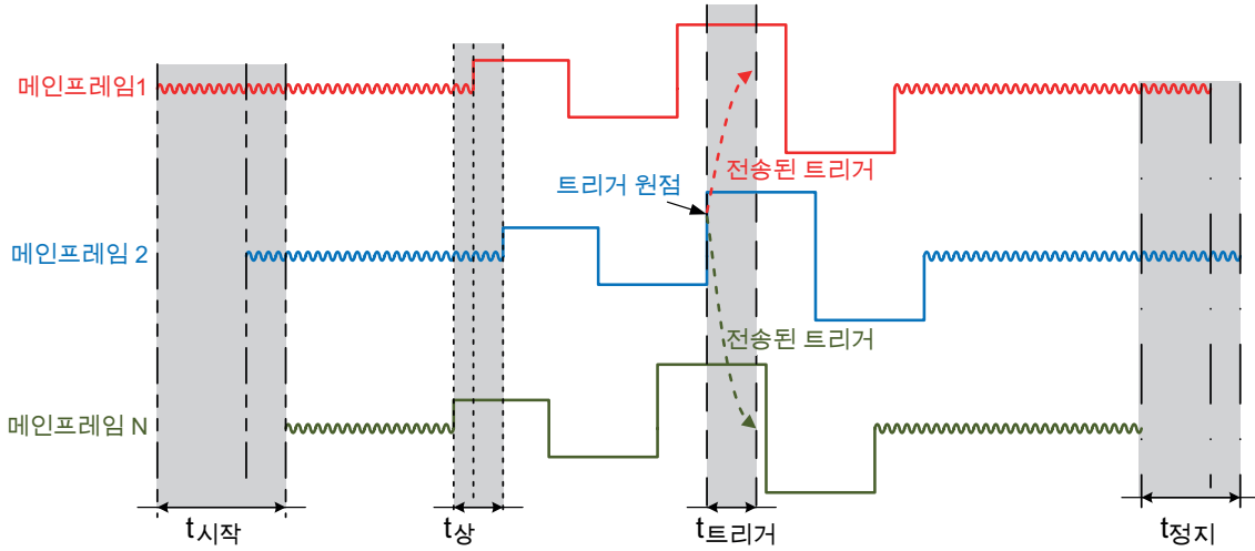
그림 13: 동기화 사양 개요
