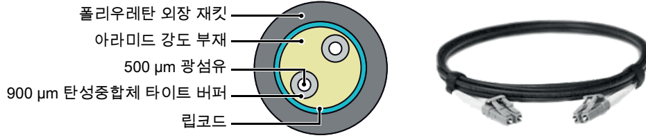
그림 24: 블록도 및 이미지
