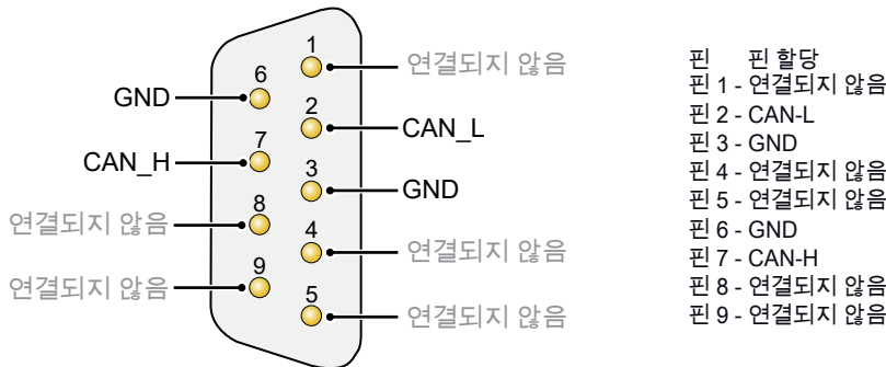
그림 32: 핀 할당 D-Sub
