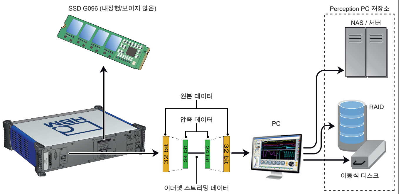
그림 11: 연속 스트리밍 개요
