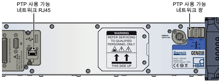
그림 10: 전기 및 광 1 Gbit 네트워크 인터페이스
