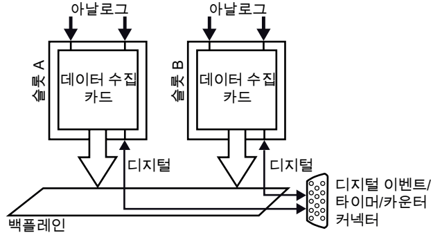
그림 15: 디지털 이벤트/타이머/카운터 블록도
