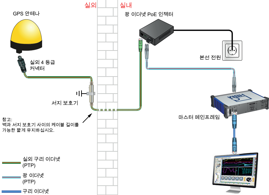
그림 28: 예제 설정 GPS 시간 동기화
