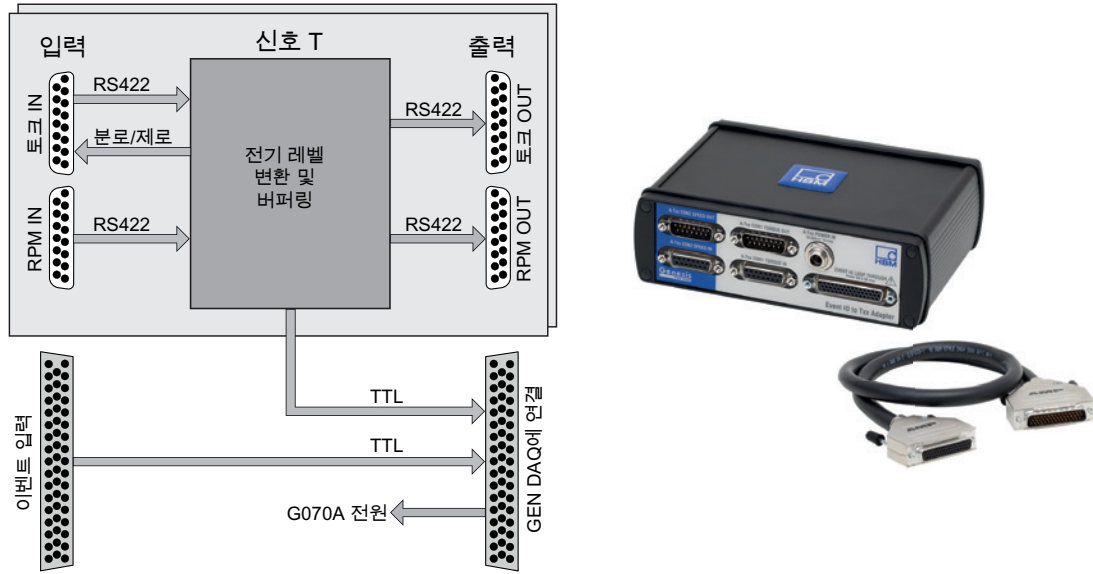
그림 25: 블록도 및 이미지
