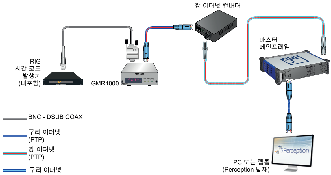
그림 27: 예제 설정 IRIG 시간 동기화
