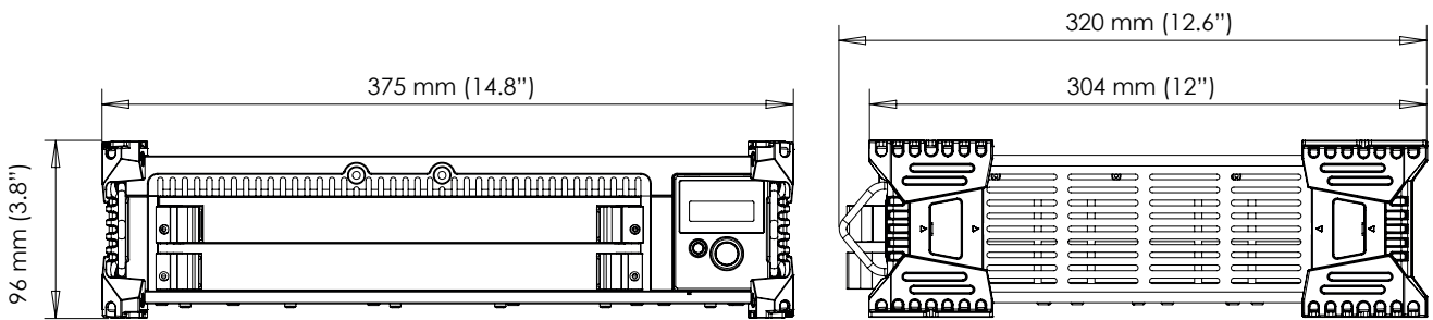
그림 1: GEN2tB 치수
