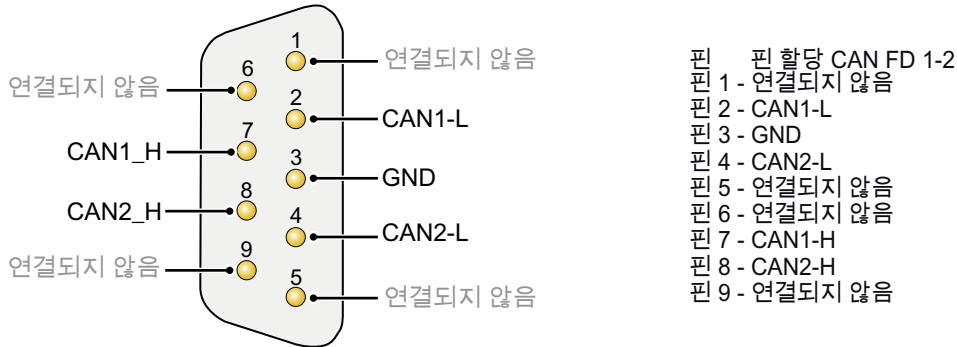
그림 30: 핀 할당 CAN FD 옵션
